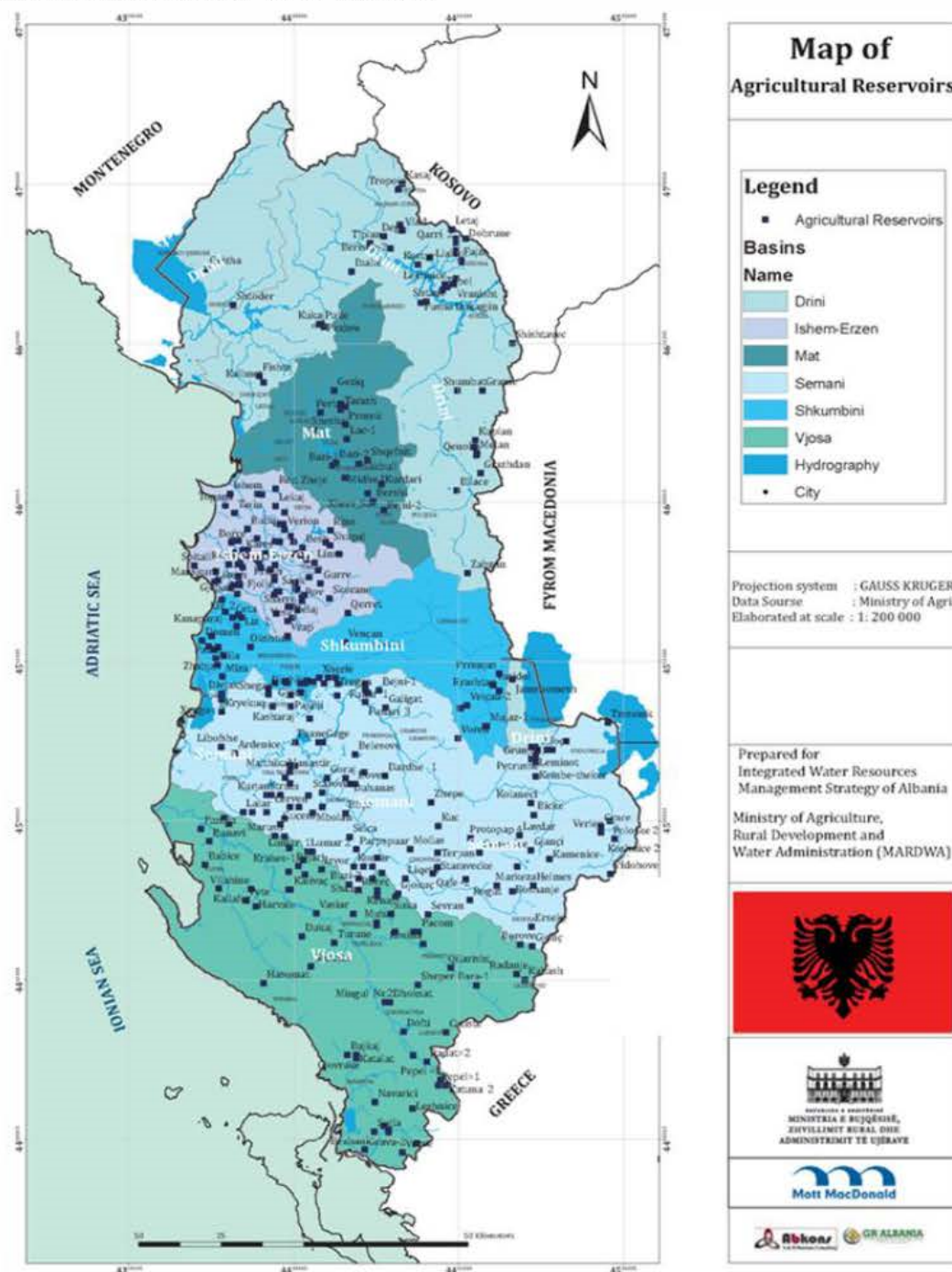
Figura 6: Vendndodhja e digave bujqësore
